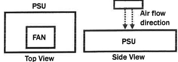
MAX Load Fan location
